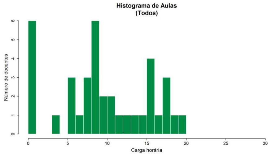
Figura 145 Histograma Total de Aulas Todos
