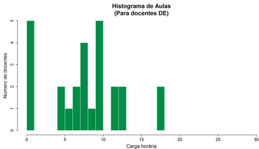
Figura 292 Histograma Total de Aulas Dedicação Exclusiva
