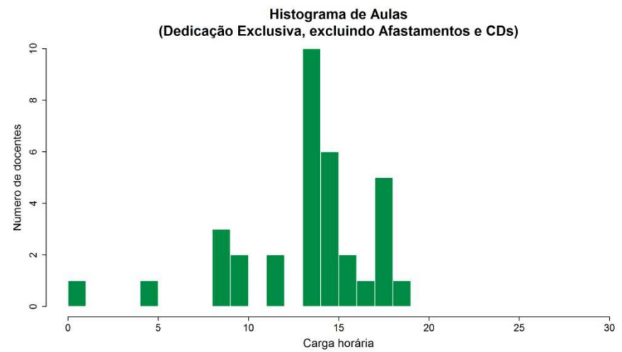
Figura 52 Histograma Total de Aulas DE, excluindo Afastamentos e CDs
