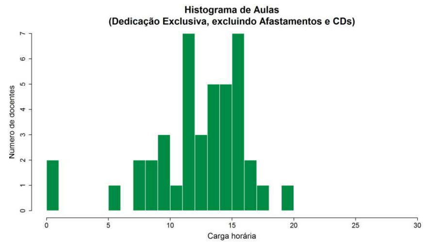
Figura 44 Histograma Total de Aulas DE, excluindo Afastamentos e CDs
