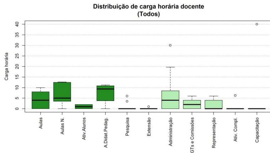
Figura 168 Boxplot Todos
