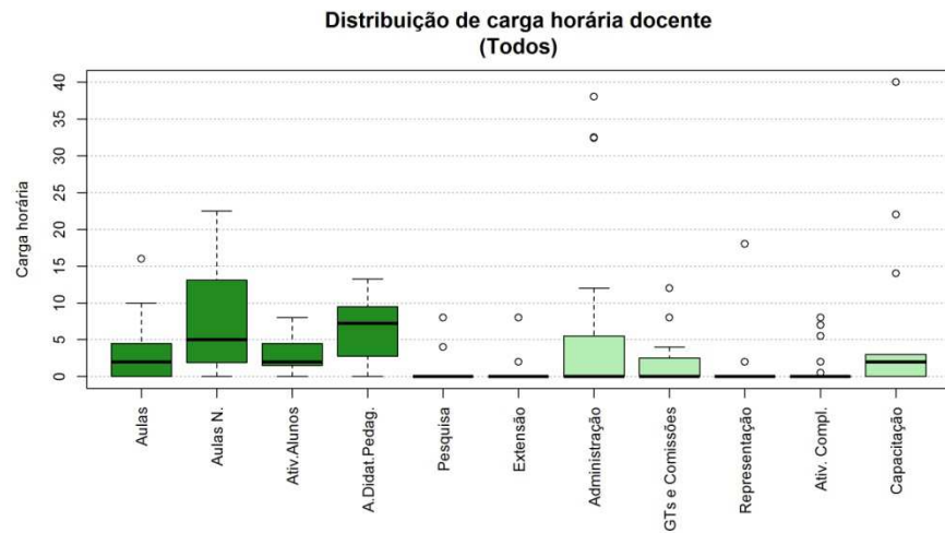
Figura 116 Boxplot Todos
