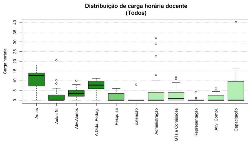
Figura 240 Boxplot Todos
