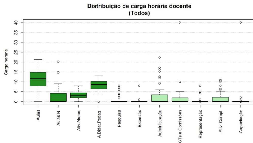
Figura 188 Boxplot Todos
