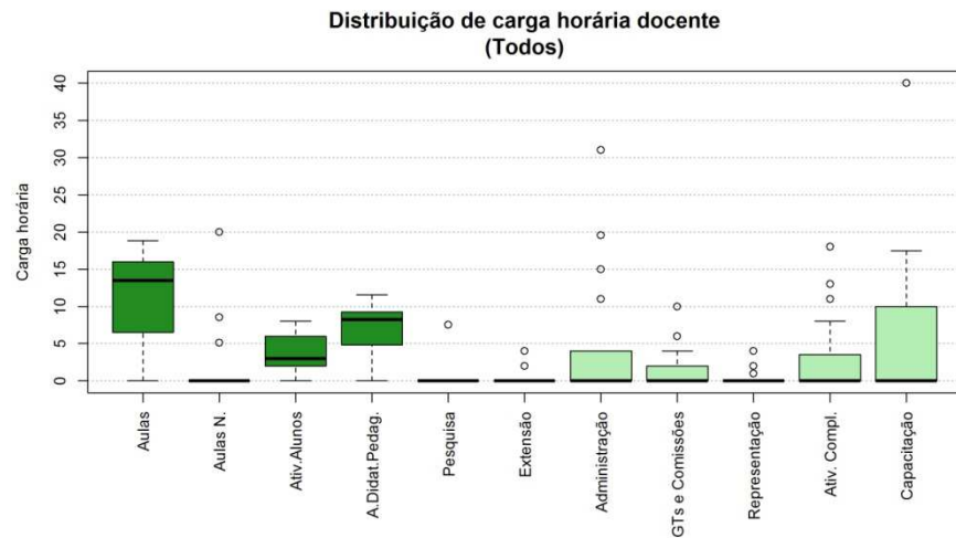
Figura 84 Boxplot Todos
