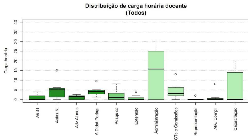
Figura 182 Boxplot Todos
