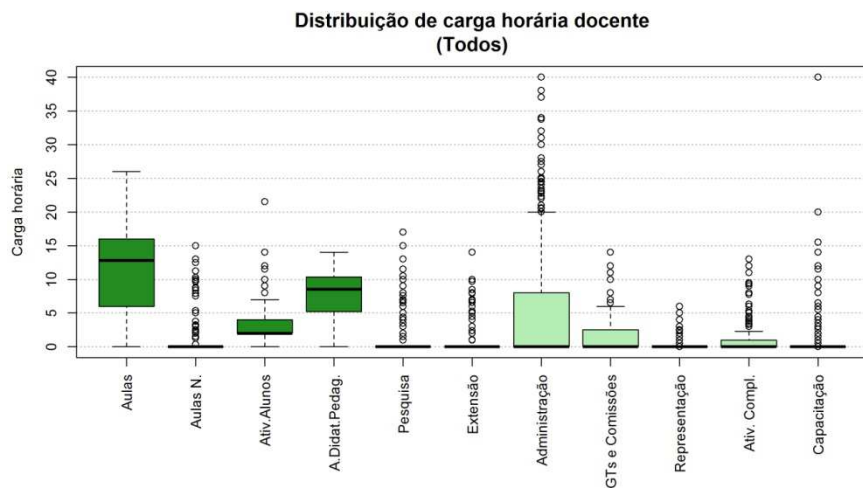
Figura 58 Boxplot Todos
