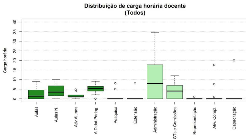
Figura 66 Boxplot Todos
