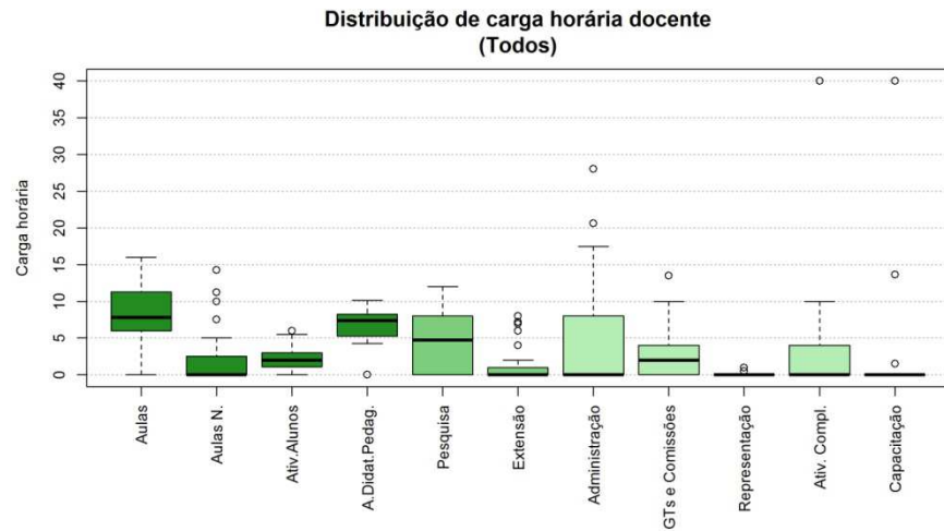
Figura 108 Boxplot Todos
