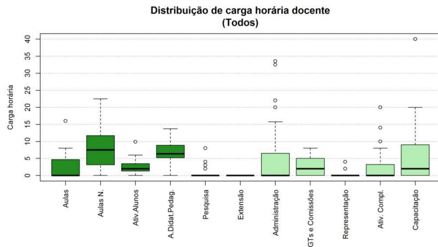
Figura 272 Boxplot Todos
