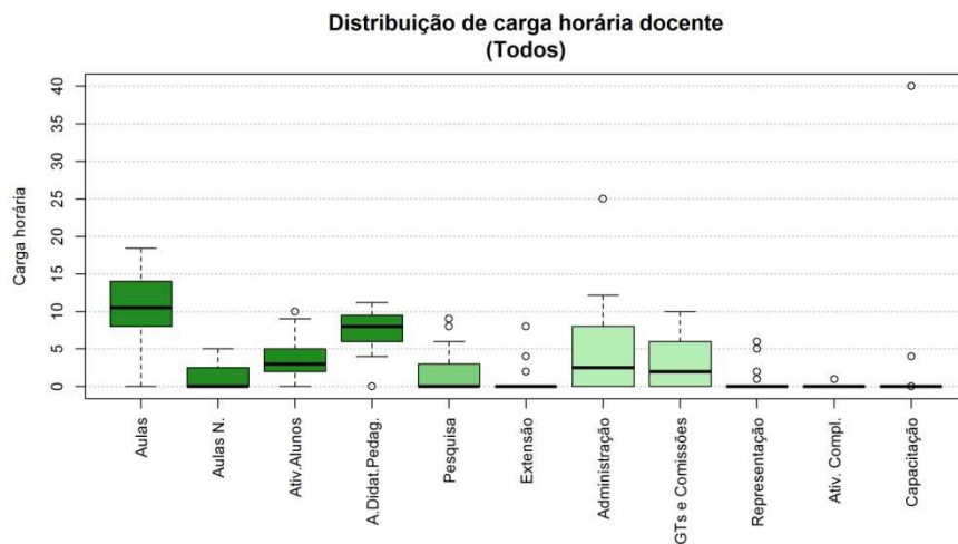
Figura 174 Boxplot Todos
