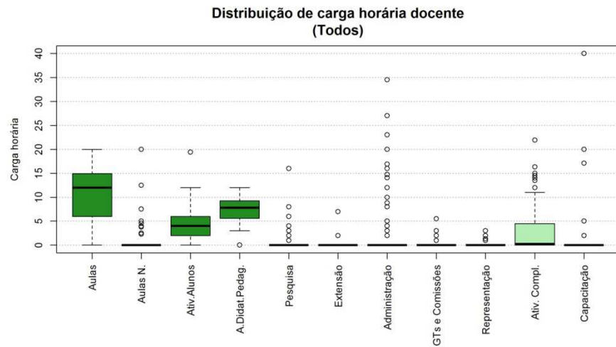
Figura 100 Boxplot Todos
