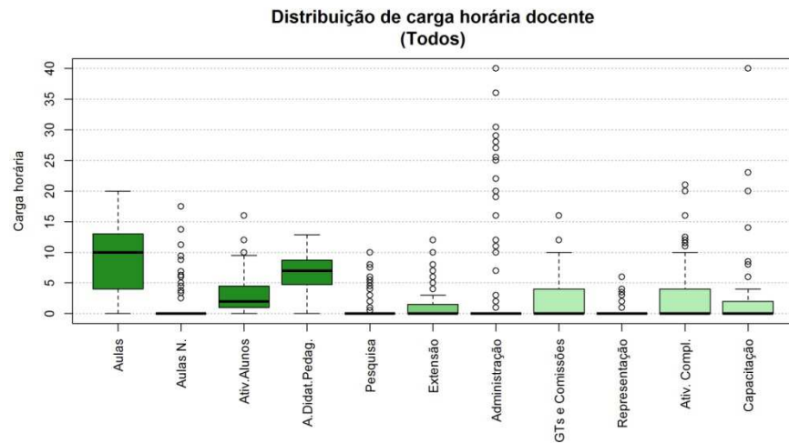
Figura 280 Boxplot Todos
