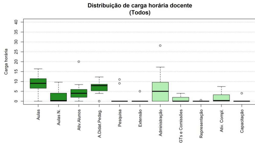
Figura 146 Boxplot Todos
