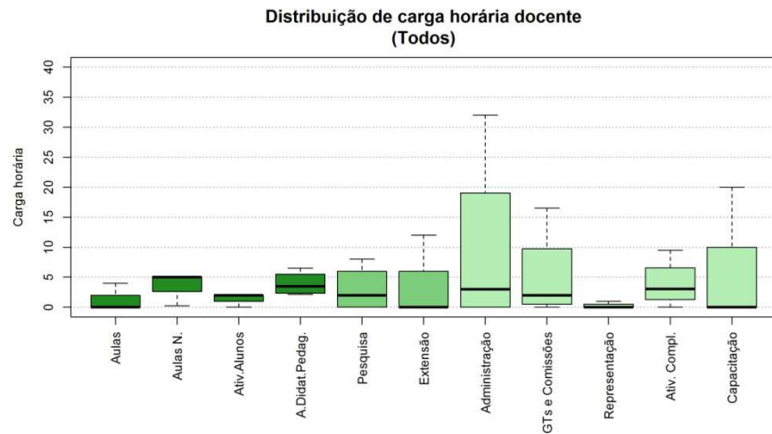
Figura 30 Boxplot Todos
