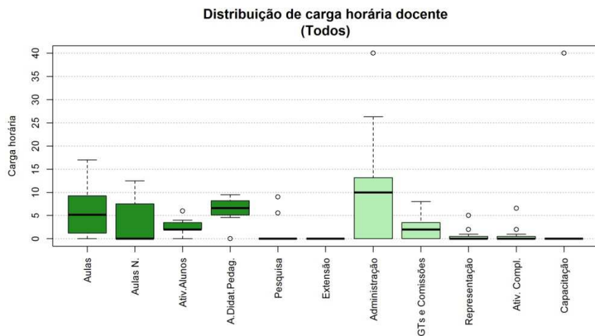
Figura 18 Boxplot Todos
