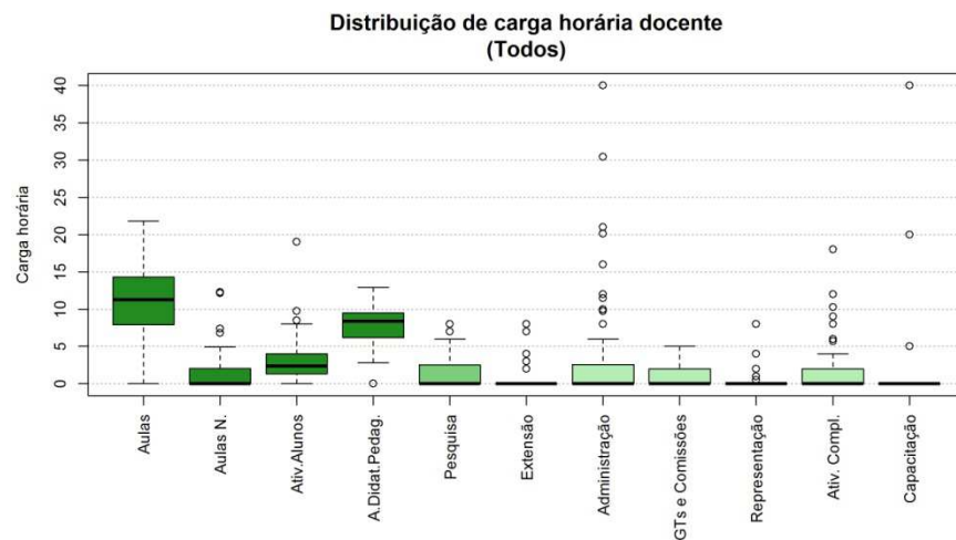
Figura 34 Boxplot Todos
