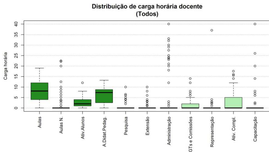
Figura 124 Boxplot Todos
