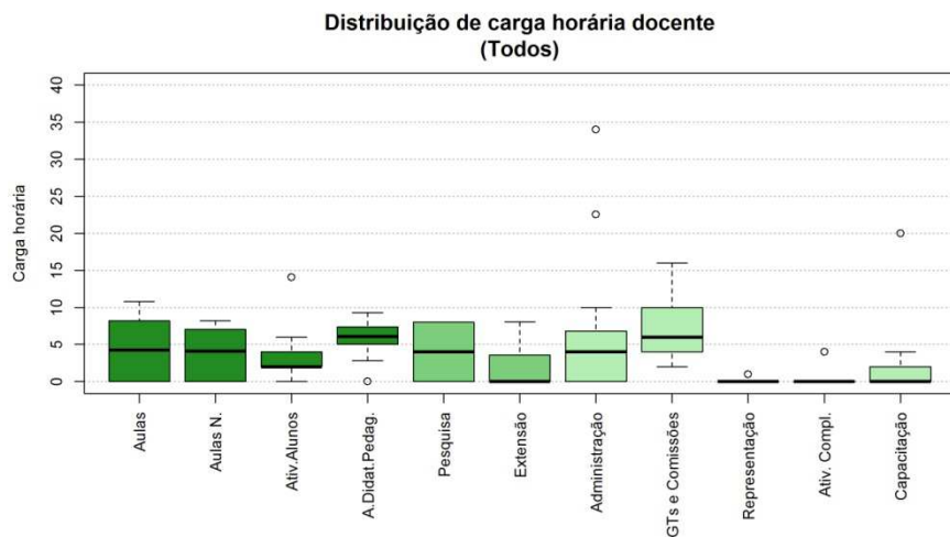
Figura 296 Boxplot Todos
