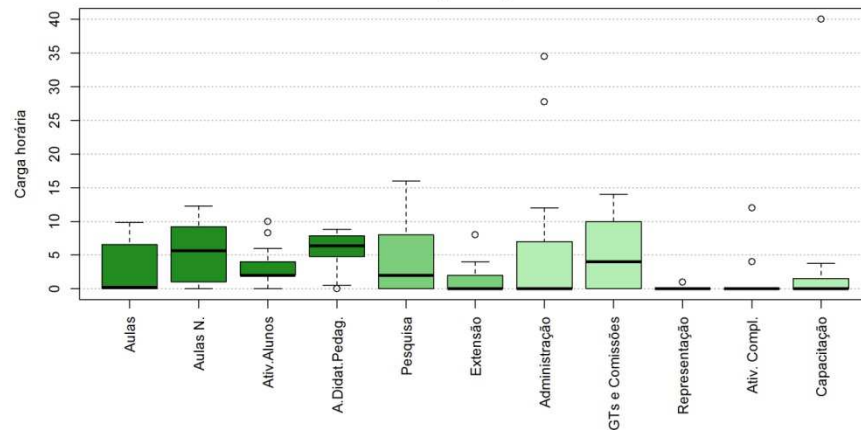
Figura 138 Boxplot Todos
