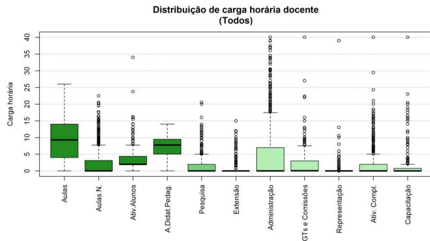
Figura 152 Boxplot Todos
