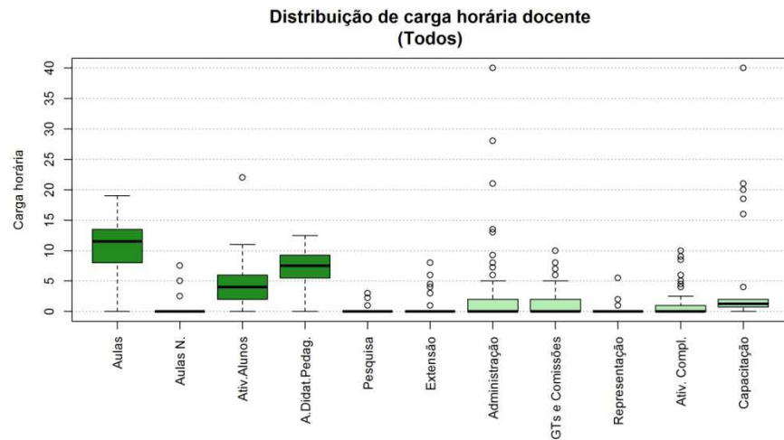
Figura 92 Boxplot Todos
