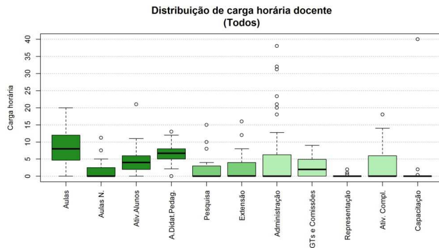
Figura 72 Boxplot Todos
