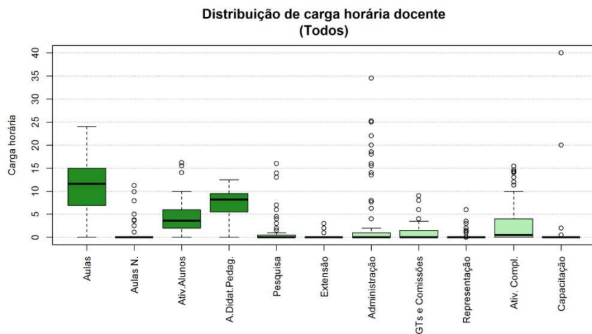
Figura 256 Boxplot Todos
