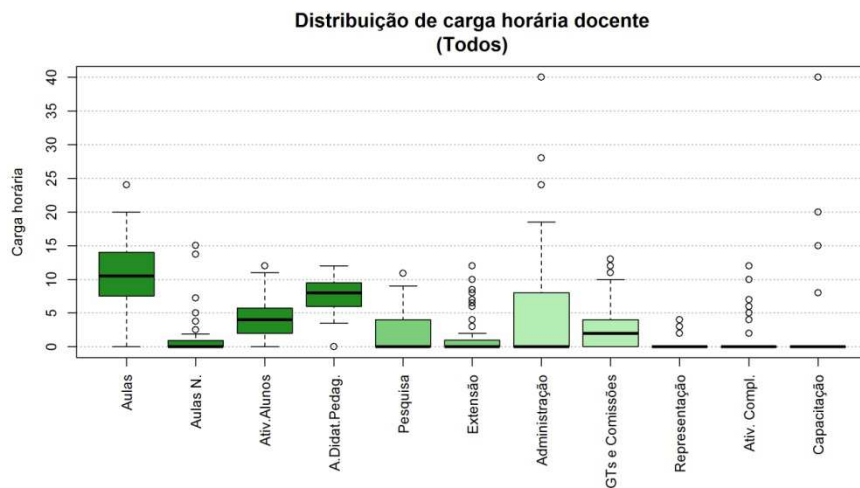
Figura 10 Boxplot Todos
