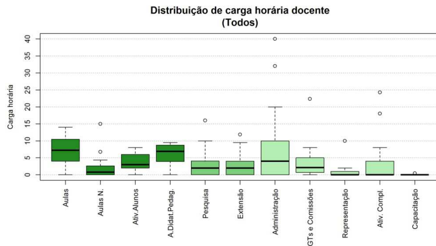
Figura 234 Boxplot Todos
