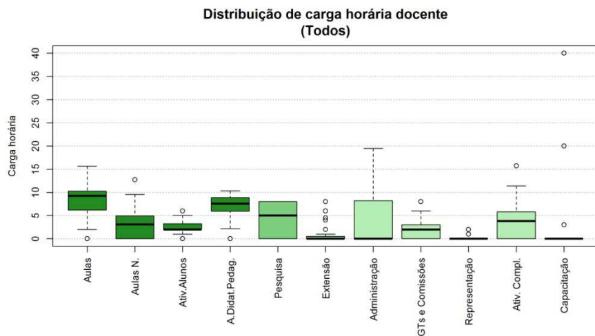
Figura 264 Boxplot Todos
