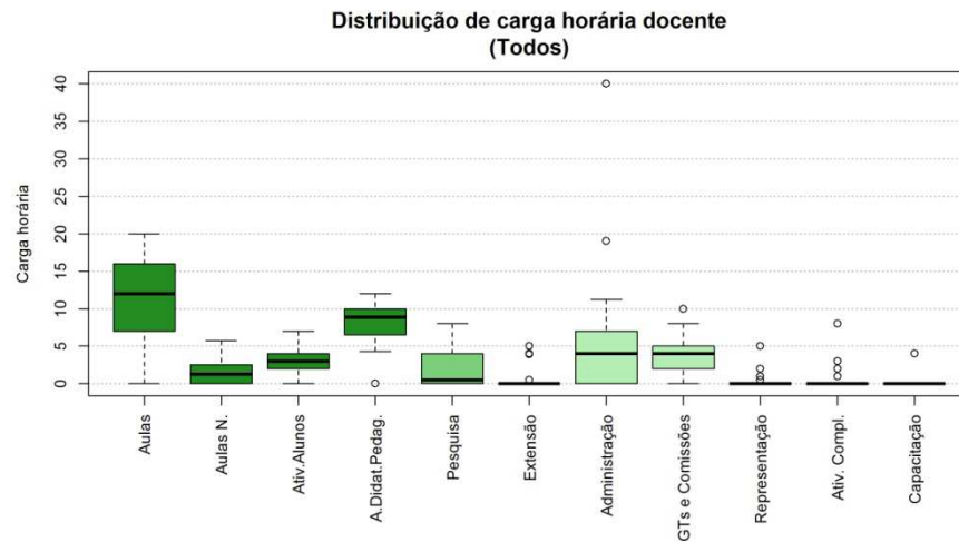
Figura 22 Boxplot Todos
