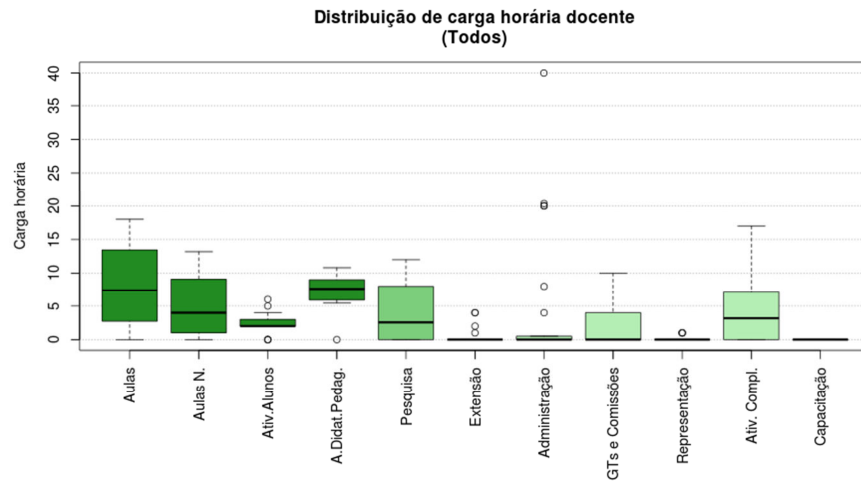
Figura 239 Boxplot Todos
