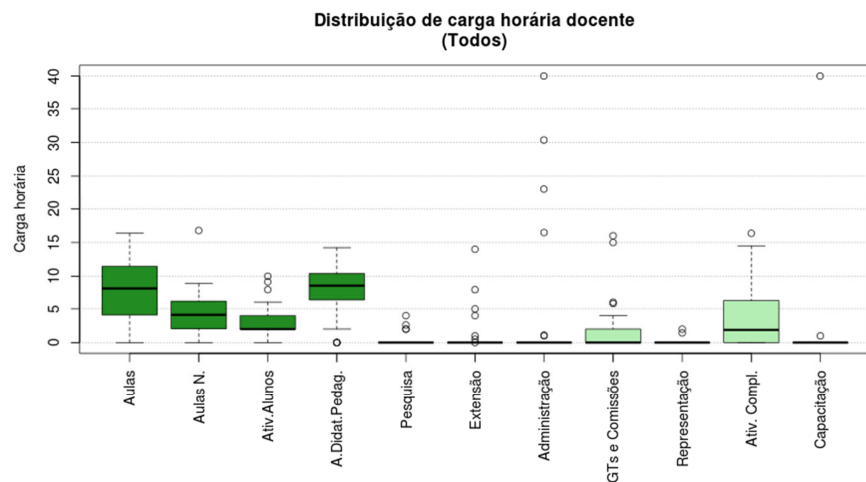
Figura 169 Boxplot Todos
