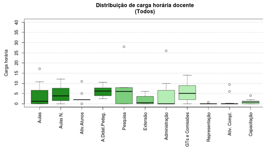
Figura 267 Boxplot Todos
