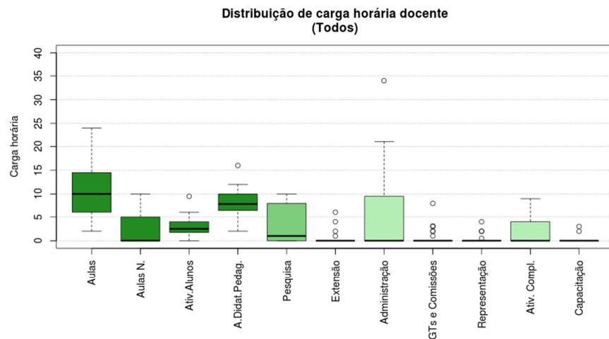
Figura 64 Boxplot Todos
