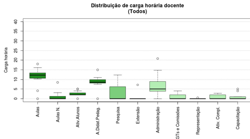
Figura 272 Boxplot Todos
