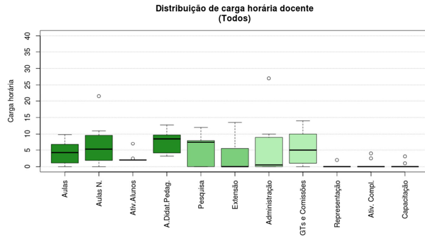
Figura 125 Boxplot Todos
