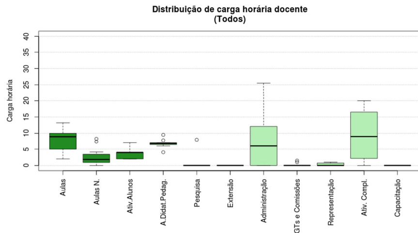
Figura 18 Boxplot Todos
