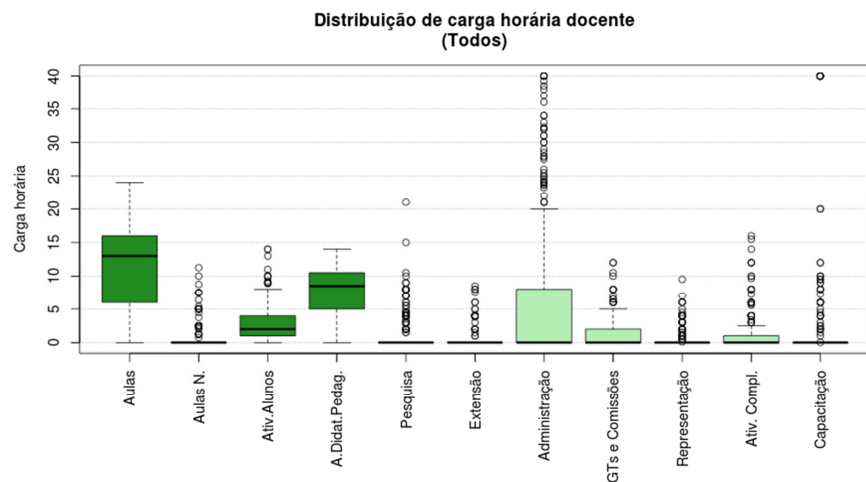
Figura 185 Boxplot Todos
