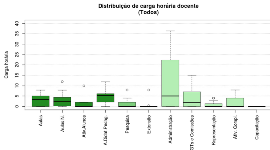
Figura 58 Boxplot Todos
