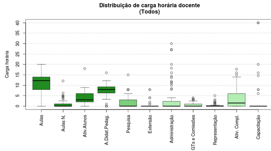
Figura 231 Boxplot Todos
