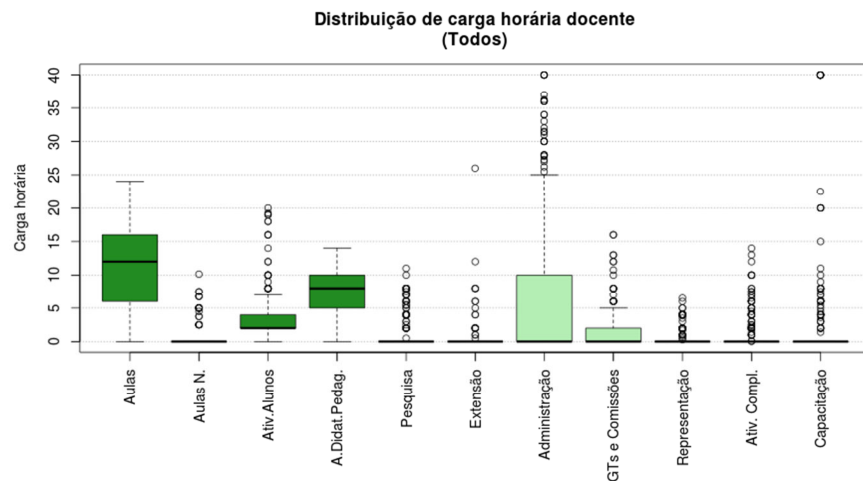
Figura 50 Boxplot Todos
