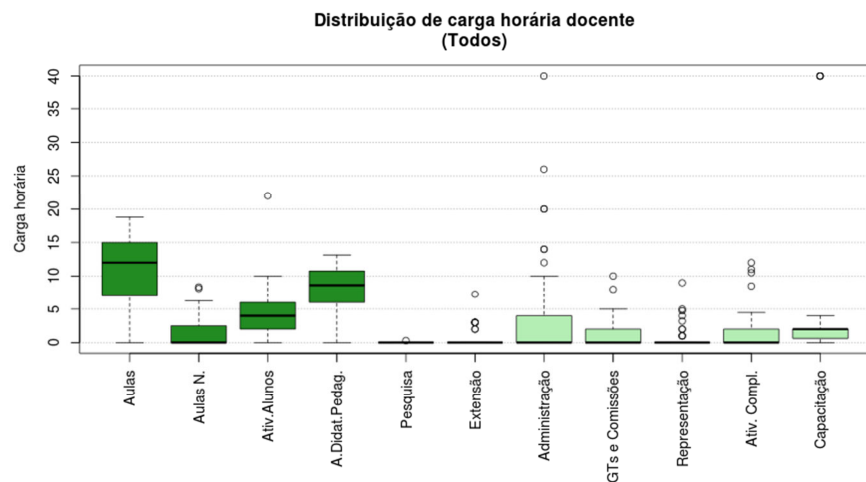
Figura 223 Boxplot Todos
