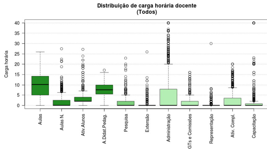
Figura 2 Boxplot Todos
