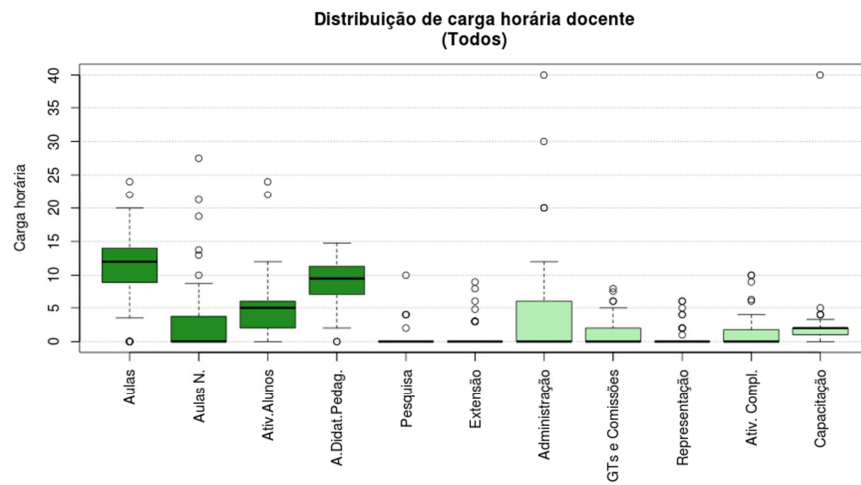
Figura 84 Boxplot Todos
