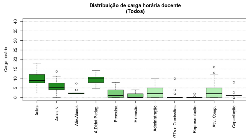
Figura 123 Boxplot Todos
