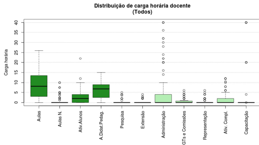
Figura 115 Boxplot Todos
