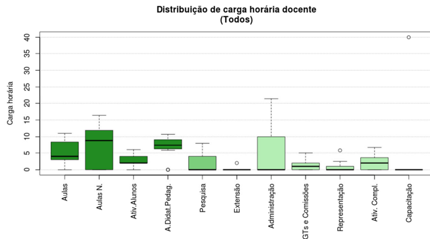
Figura 149 Boxplot Todos
