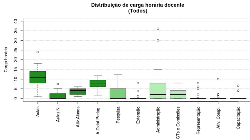
Figura 153 Boxplot Todos
