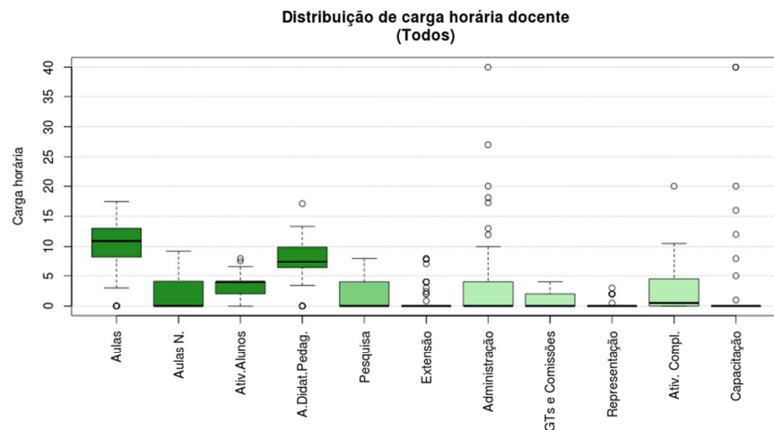
Figura 26 Boxplot Todos
