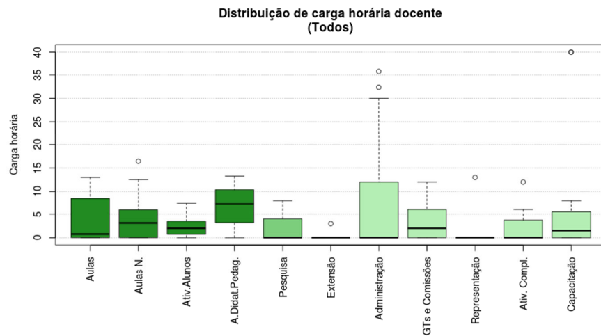
Figura 245 Boxplot Todos
