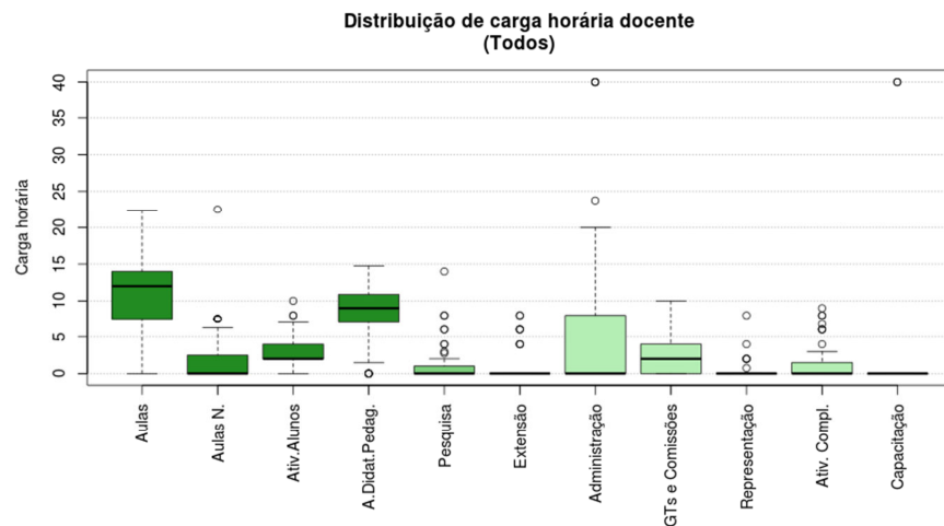
Figura 10 Boxplot Todos
