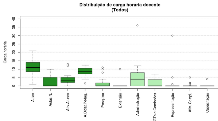
Figura 20 Boxplot Todos
