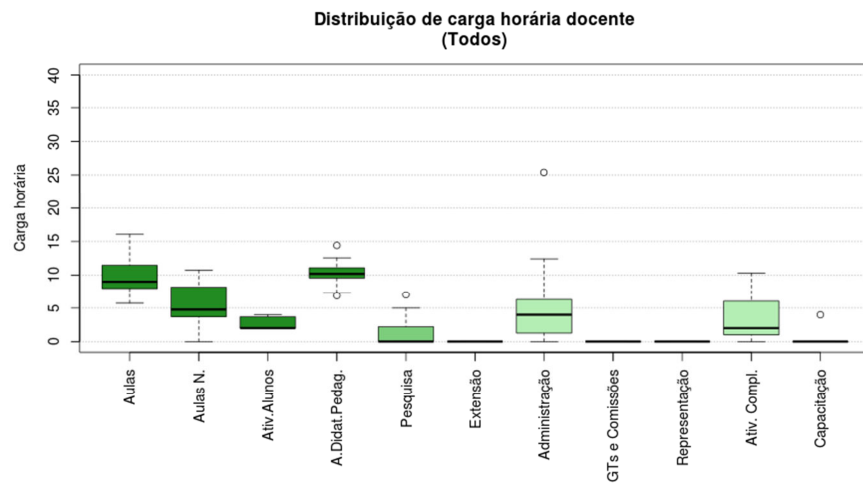
Figura 131 Boxplot Todos
