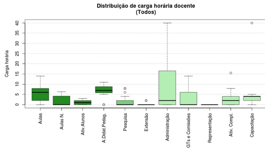
Figura 107 Boxplot Todos
