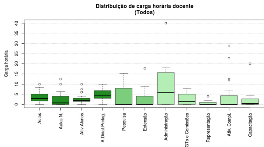
Figura 207 Boxplot Todos
