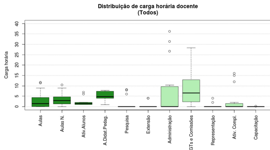
Figura 193 Boxplot Todos
