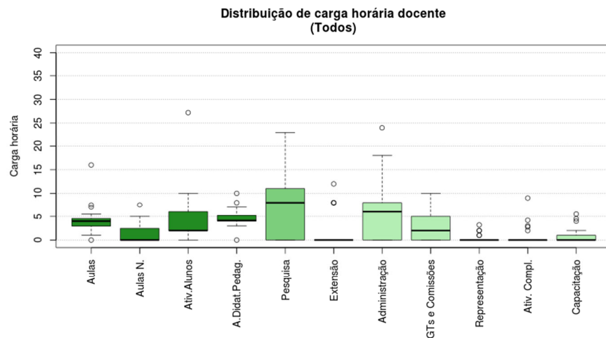
Figura 72 Boxplot Todos
