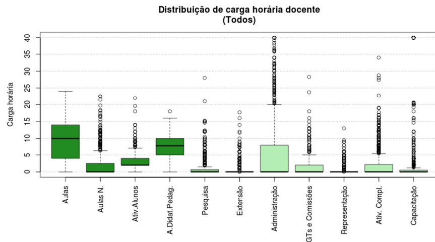
Figura 133 Boxplot Todos
