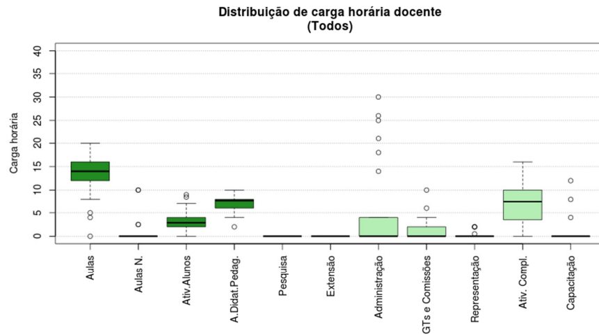
Figura 76 Boxplot Todos
