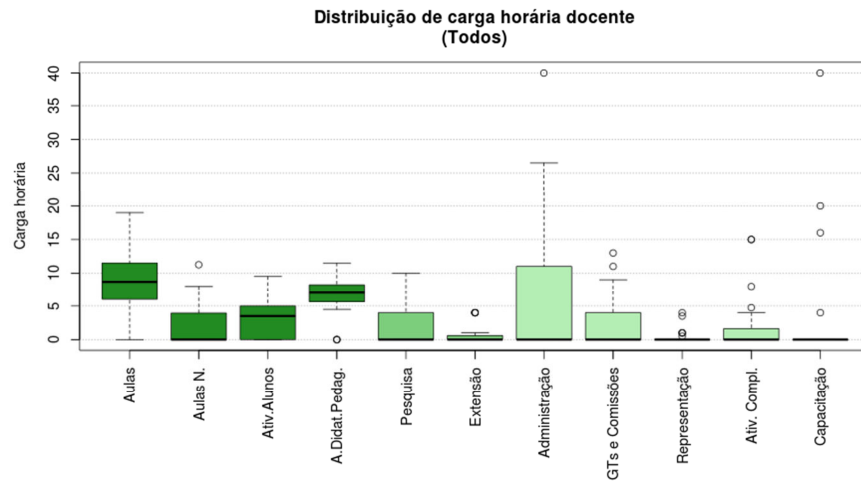
Figura 199 Boxplot Todos
