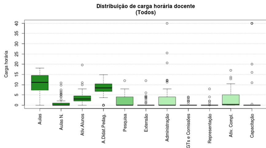
Figura 161 Boxplot Todos
