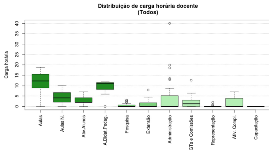
Figura 34 Boxplot Todos
