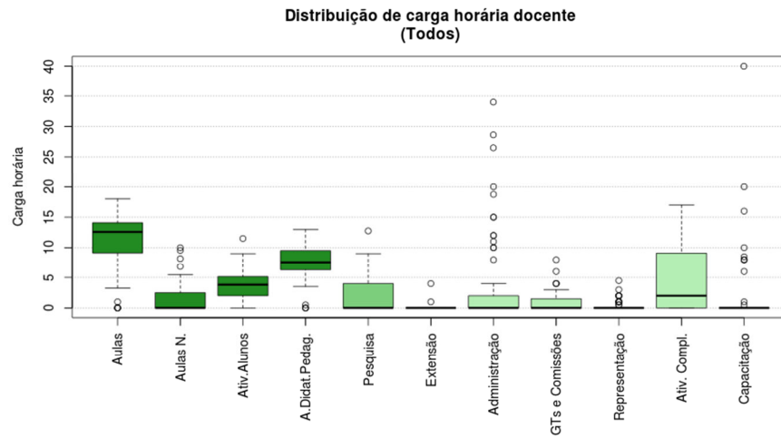
Figura 92 Boxplot Todos
