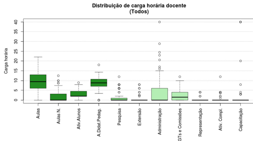
Figura 141 Boxplot Todos
