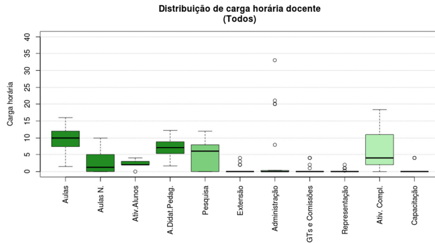
Figura 100 Boxplot Todos
