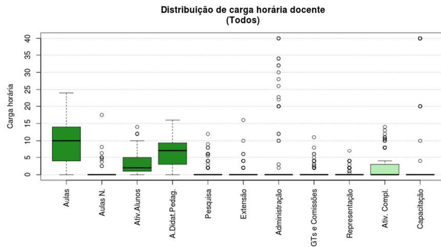
Figura 253 Boxplot Todos
